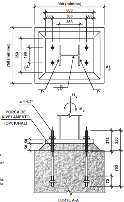
CORTE A-A
