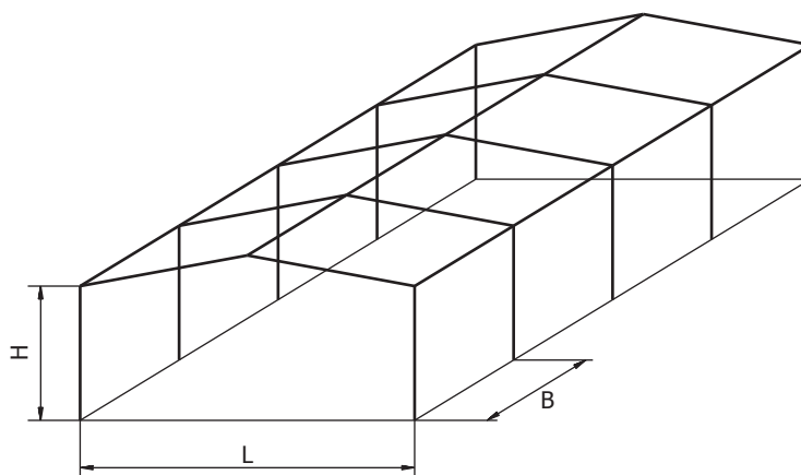
Figura 1 - Dimensões Padrão
