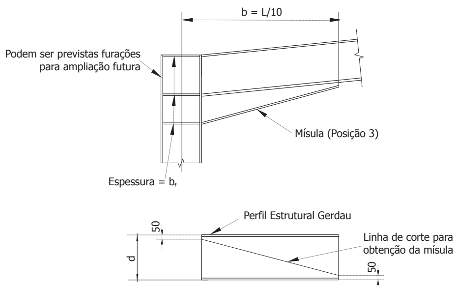
Figura 8 - Nó do Pórtico e Recorte das Mísulas
