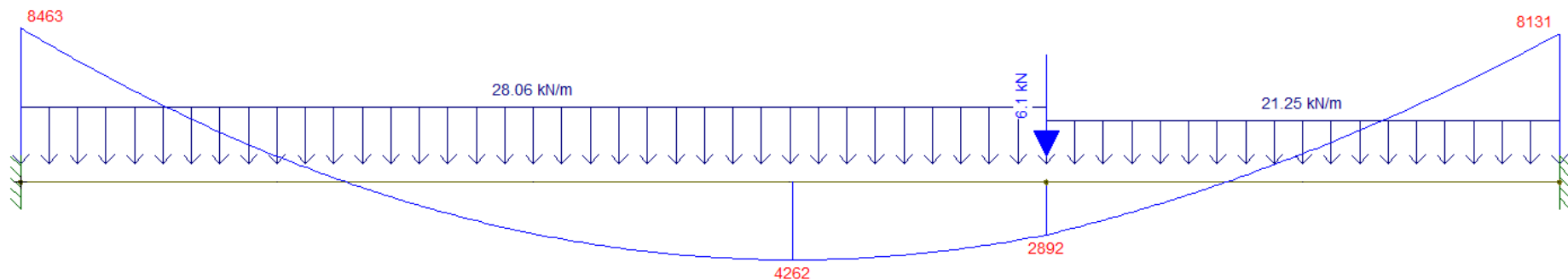
Momento Fletor
