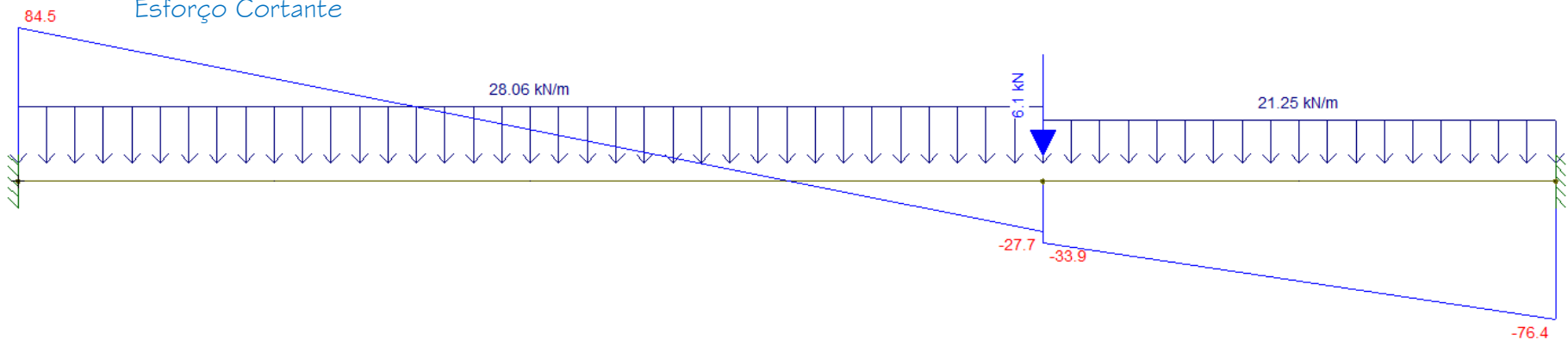
Esforço Cortante
