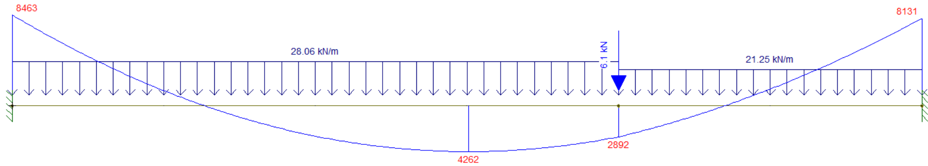
Momento Fletor
