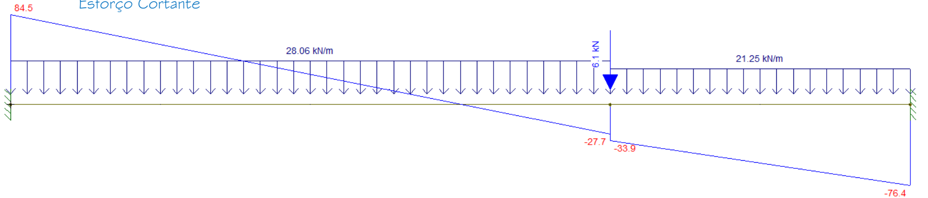
Esforço Cortante
